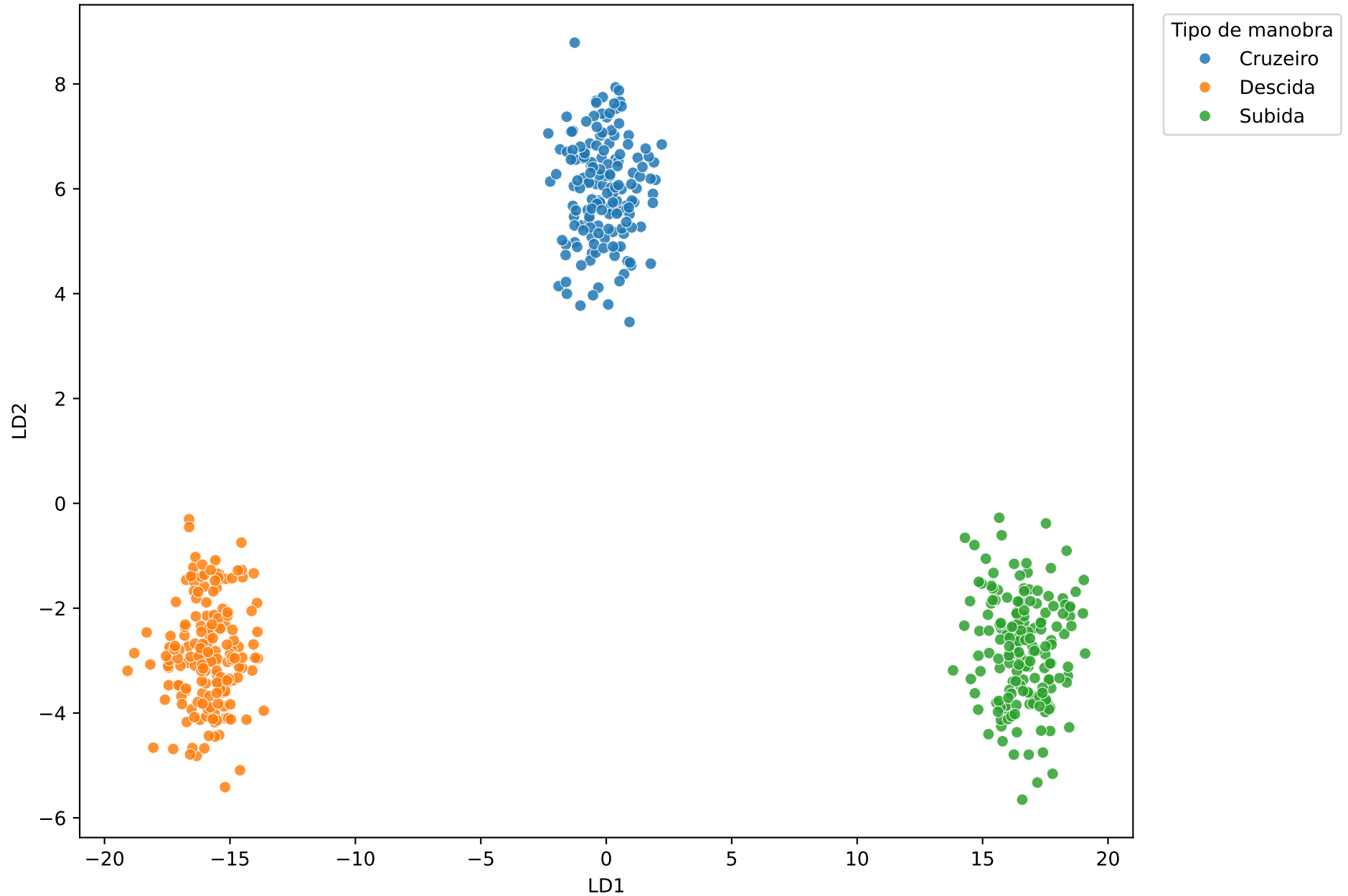
Visualização LDA 2D — usa o rótulo tipo_manobra
